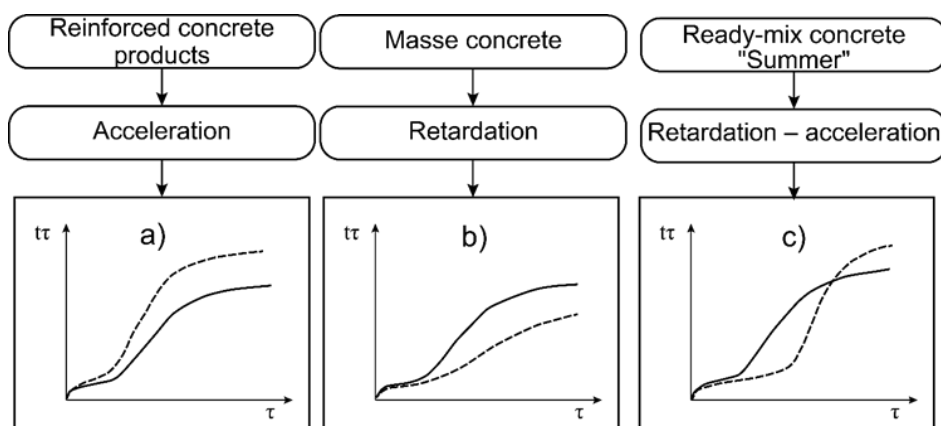
Rys. 5. Funkcjonalno-kinetyczne schematy wpływu dodatków.
