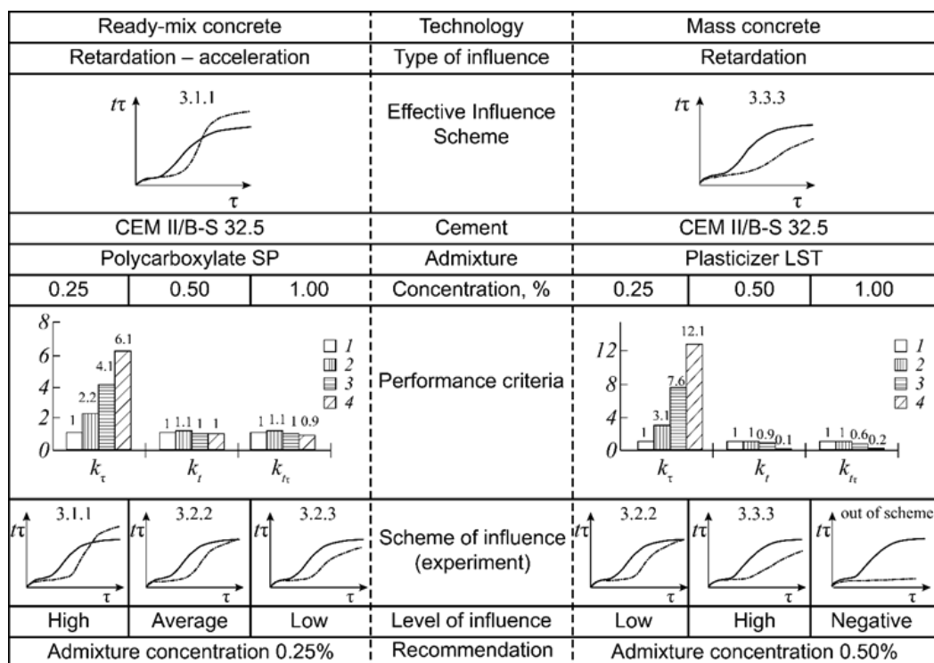
Rys. 7. Monitorowanie funkcjonalno-kinetyczne wpływu uplastyczniaaczy na twardnienie betonu.
